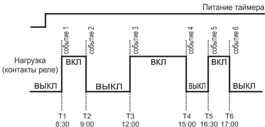
Рисунок 3.5 – Включение нагрузки на примере суточного режима работы
