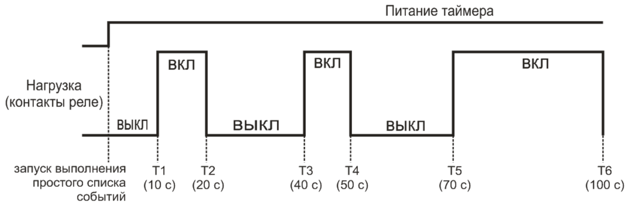
Рисунок 3.6 – Включение нагрузки на примере простого режима работы
