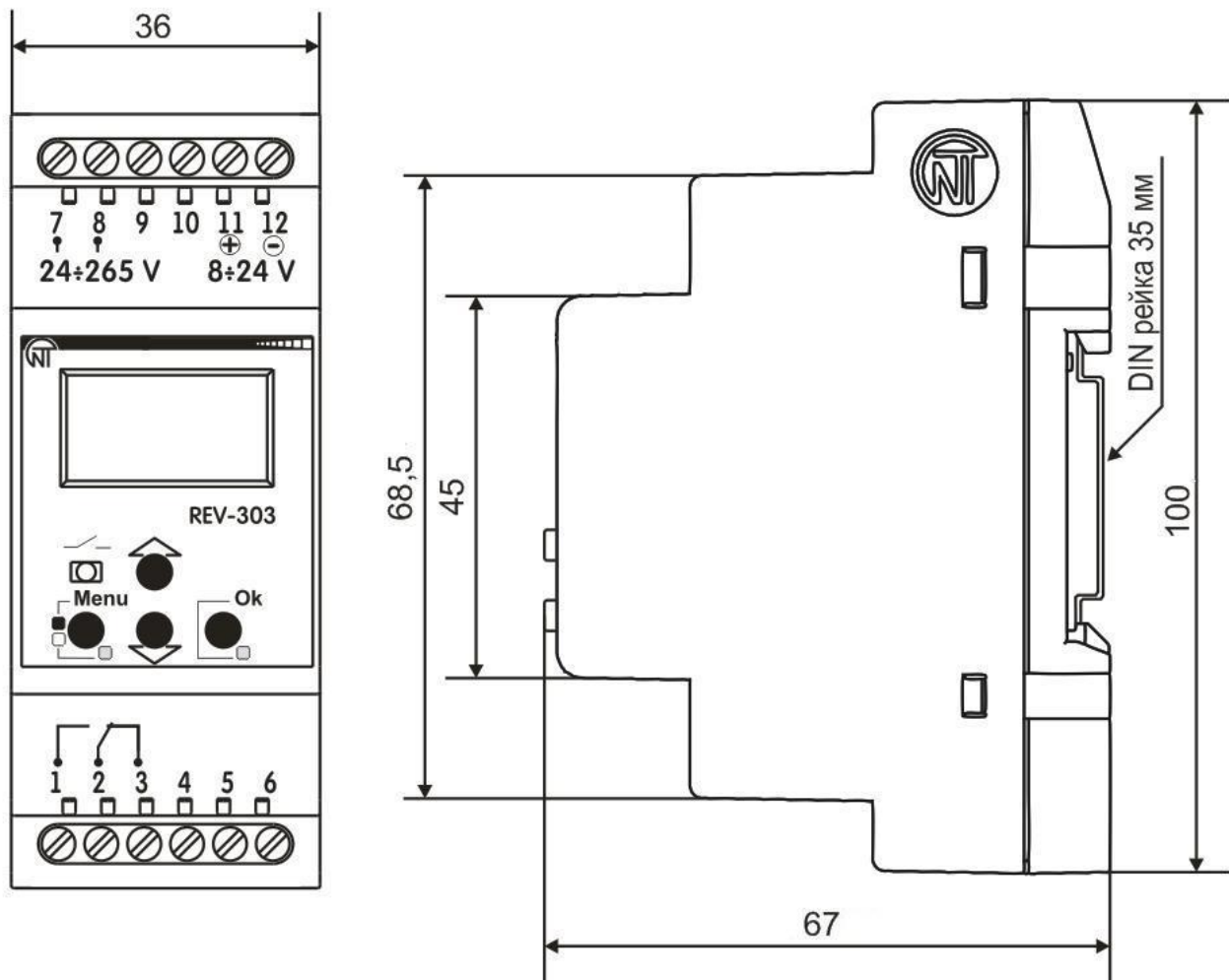
Рисунок 3.1 – Внешний вид и габаритные размеры таймера
