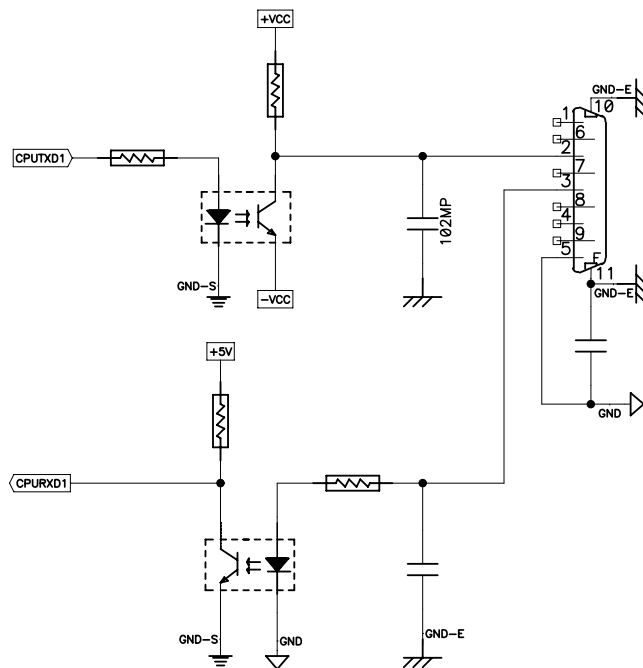
Рис. 11: Последовательный интерфейс DB9
